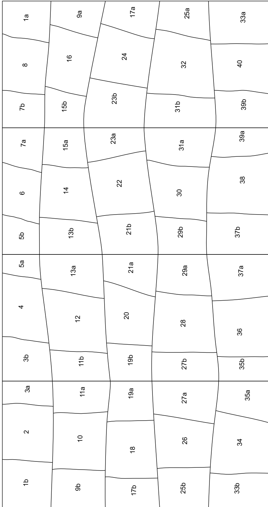
Schnittmuster Übersicht im Maßstab 1:3
